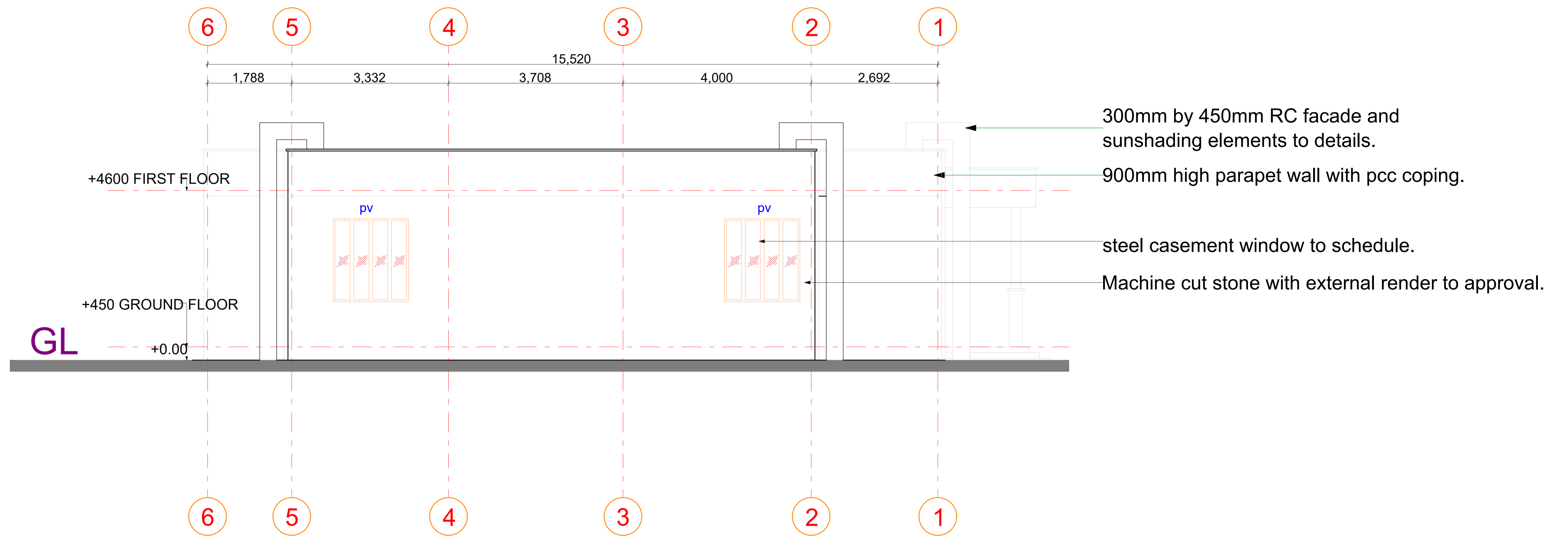
ELEVATION 07
