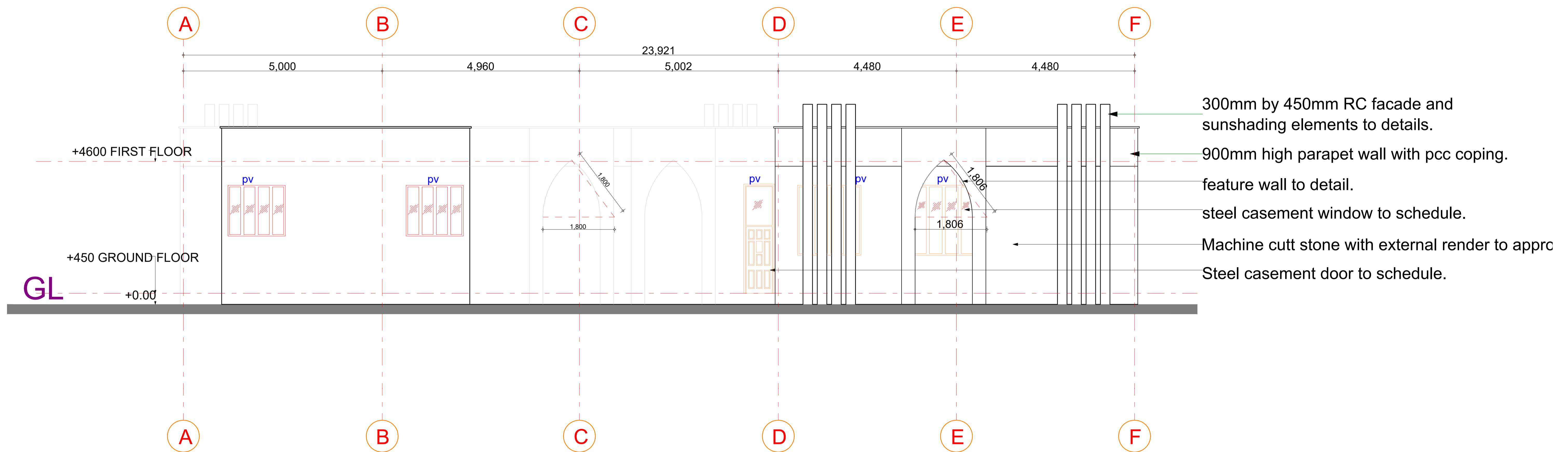
ELEVATION 08
