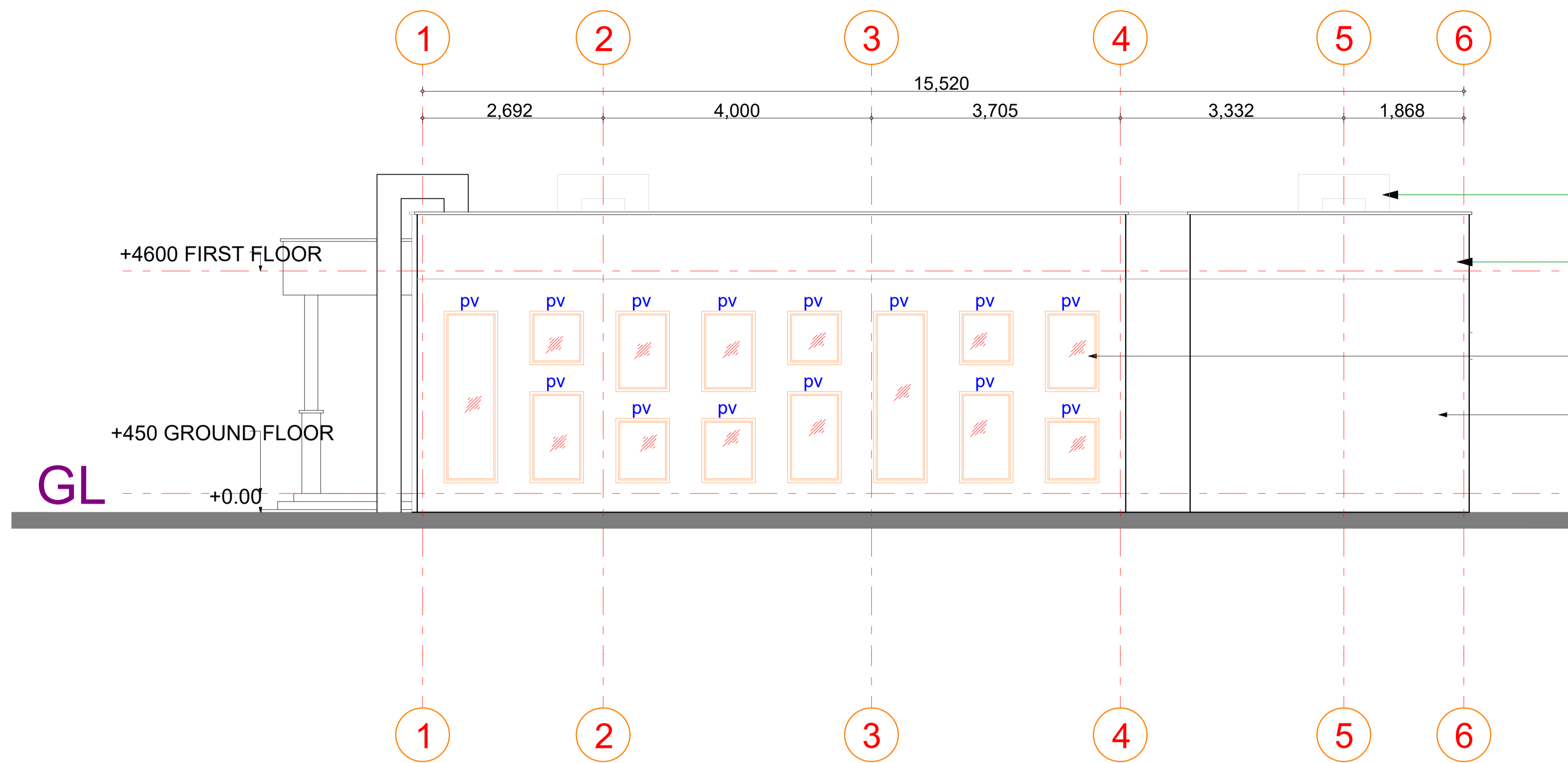
ELEVATION 05
