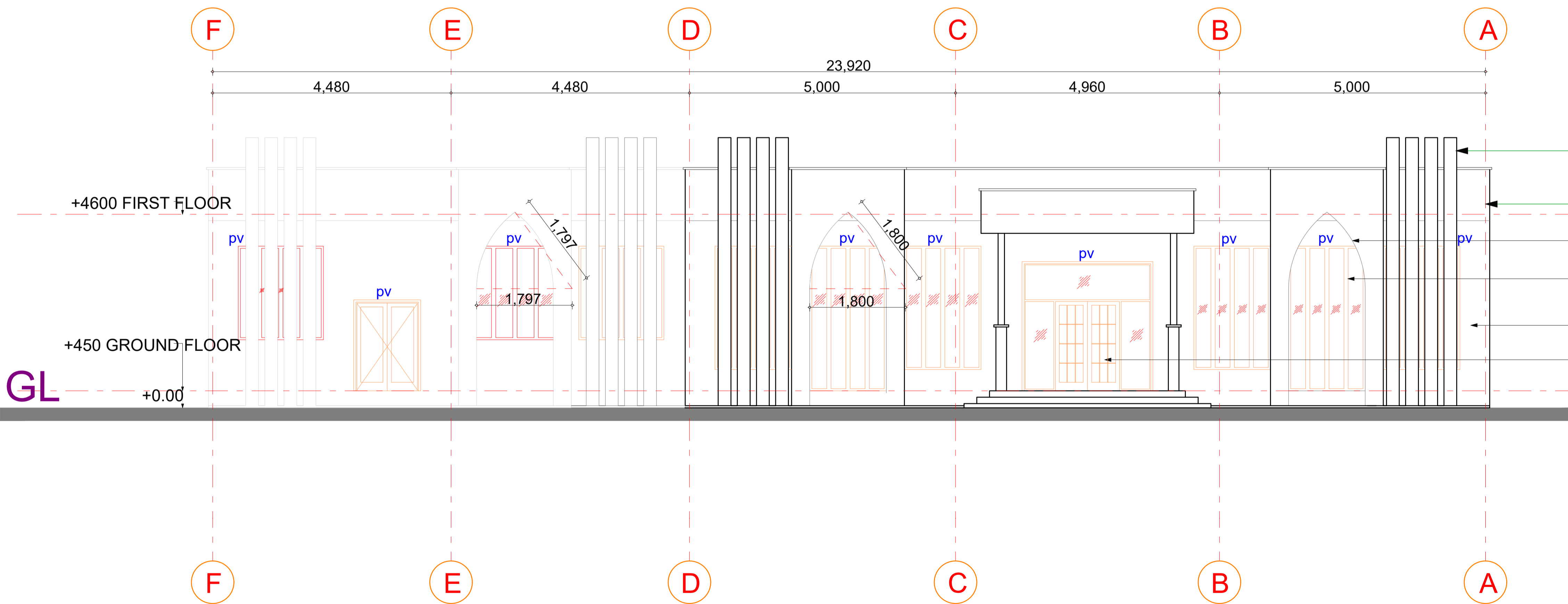
ELEVATION 06
